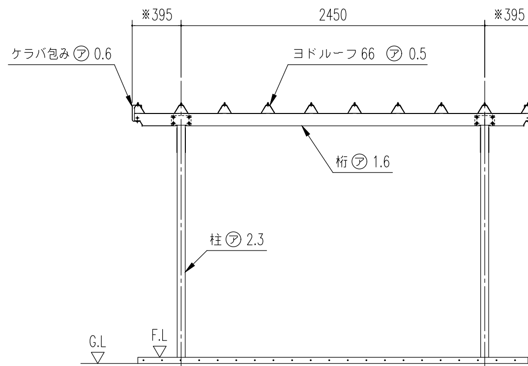
正面断面図 (S= 1/30)
