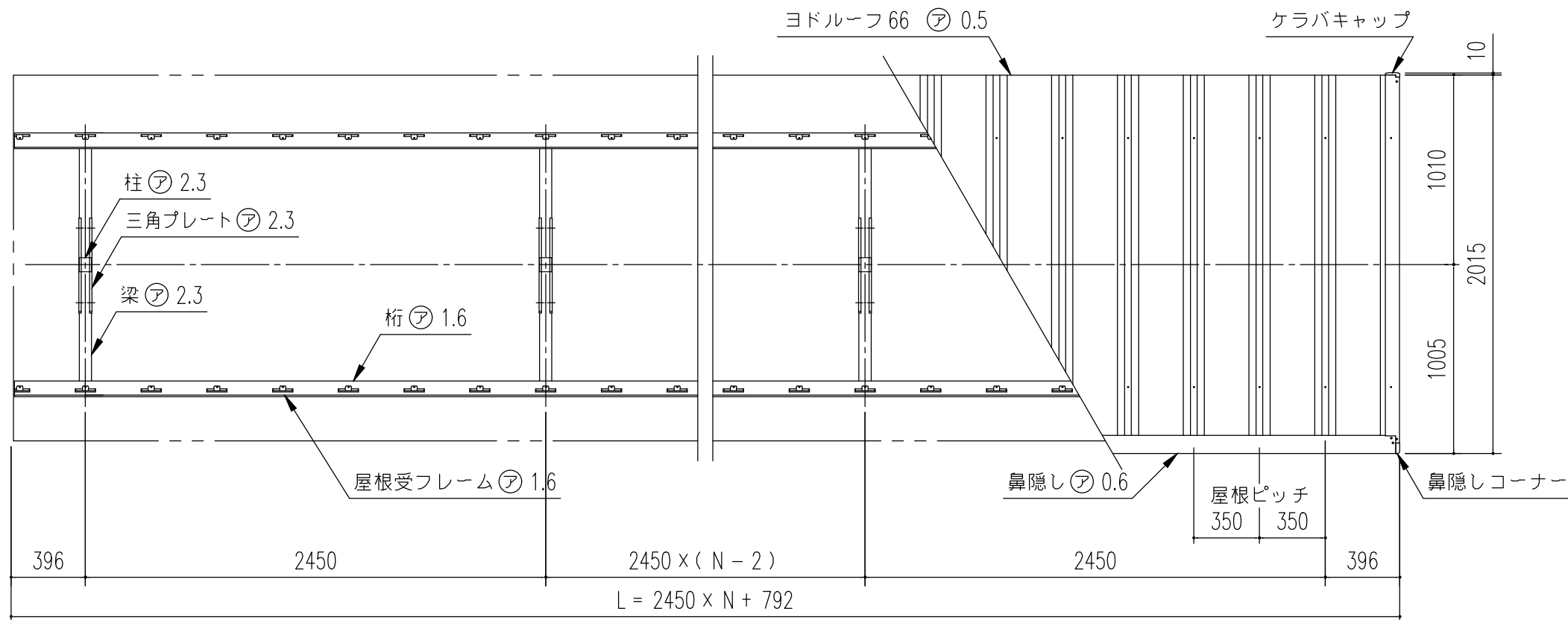
小屋伏図 (S=1/30)
