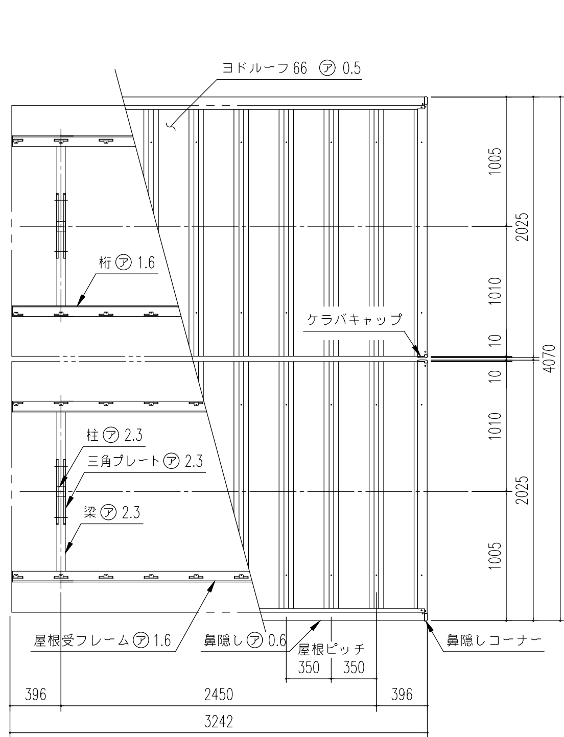
小屋伏図 (S= 1/30)
