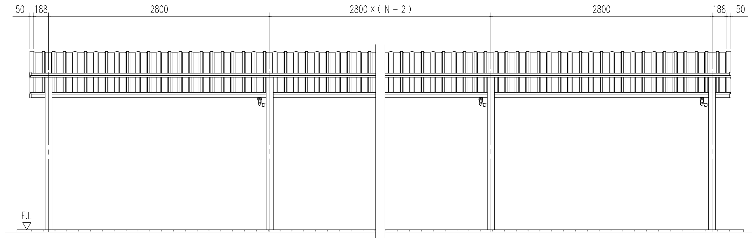
正面立面図 (S= 1/30) ( N : スパン数 )
