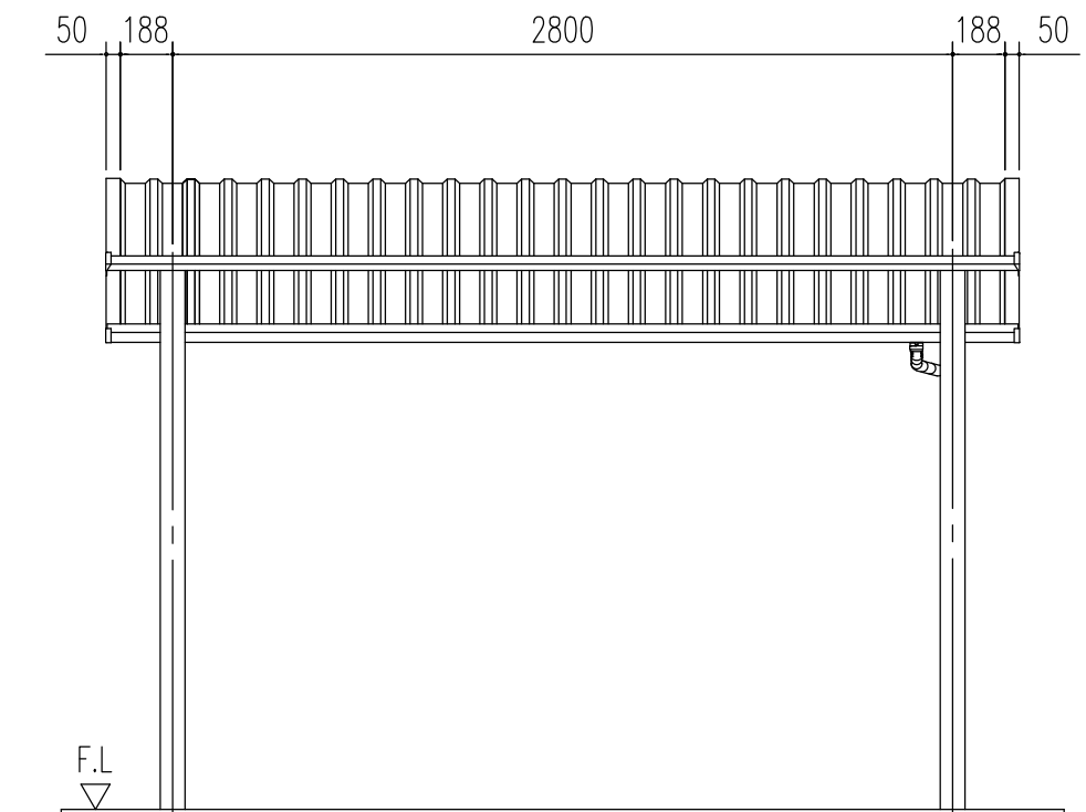
正面立面図 (S= 1/30)
