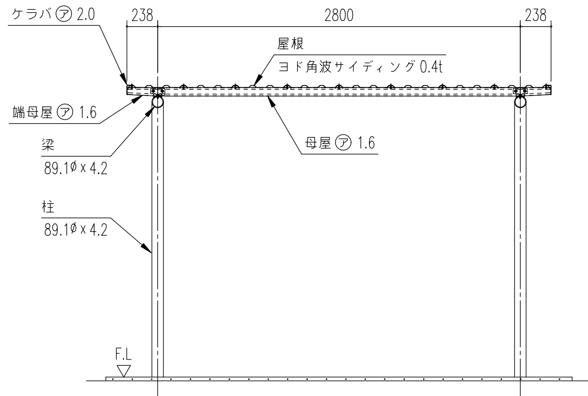
正面断面図 (S= 1/30)
