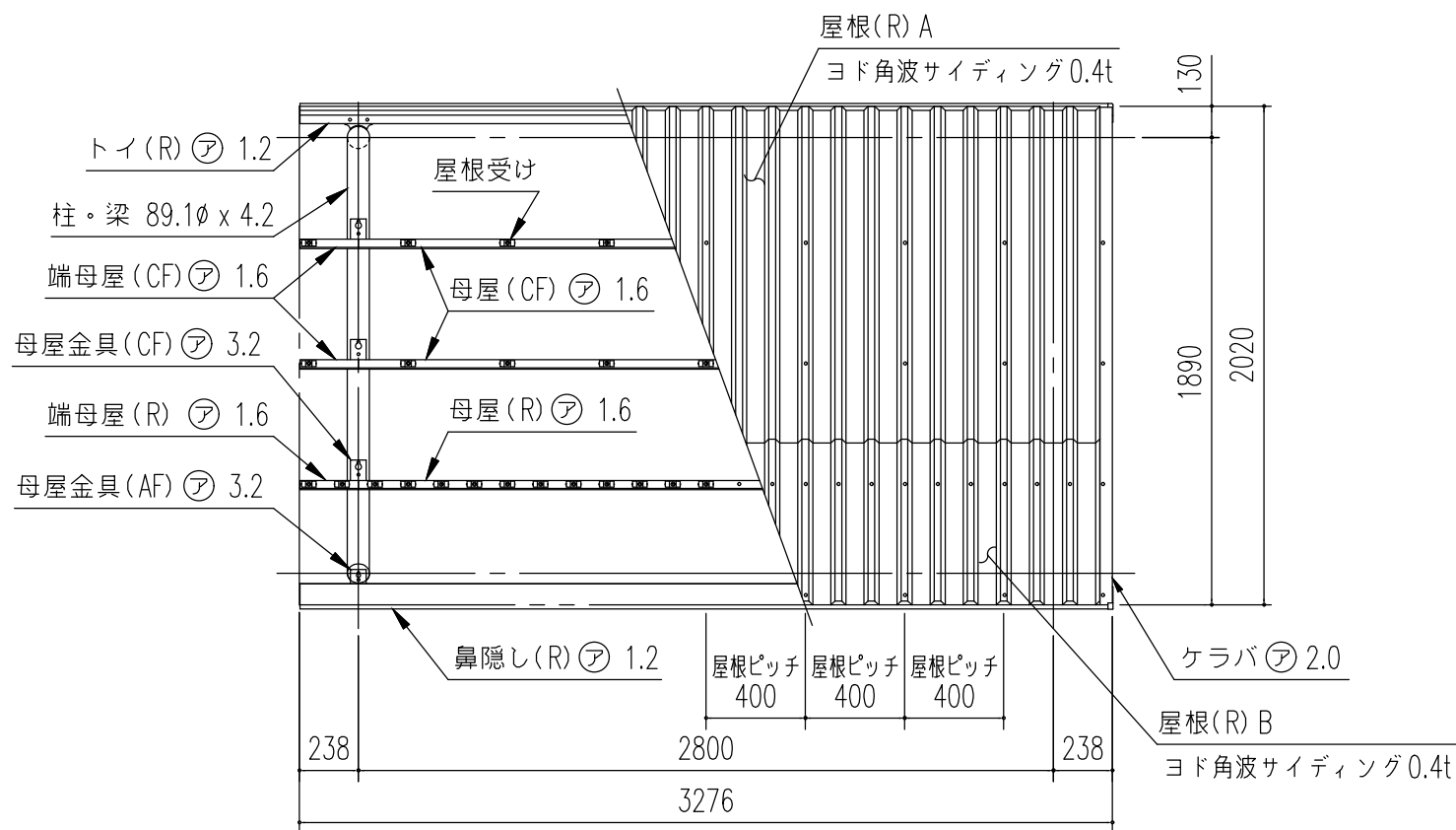
小屋伏図 (S= 1/30)
