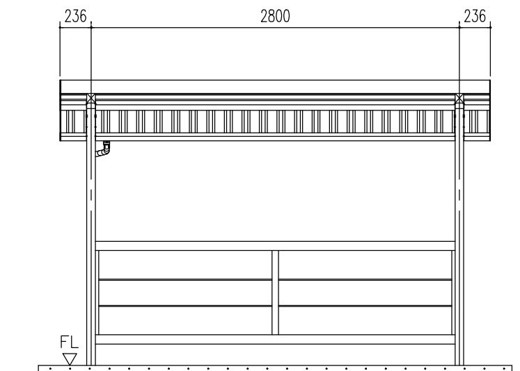
正面立面図 (S=1/40)
