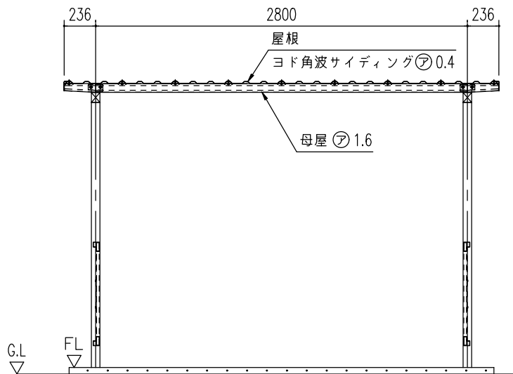
正面断面図 (S= 1/40)
