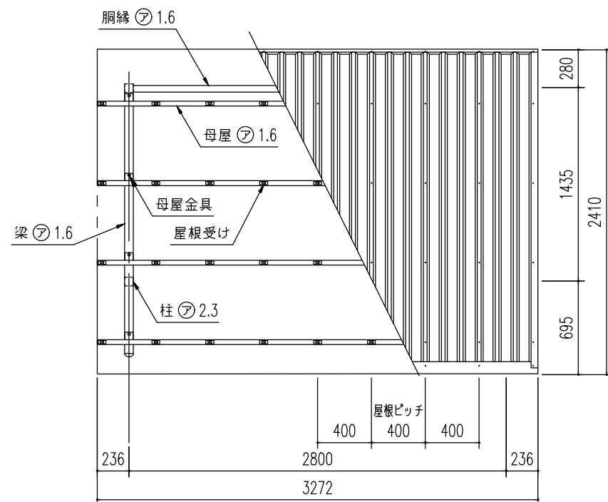
小 屋 伏 図 (S= 1/40)
