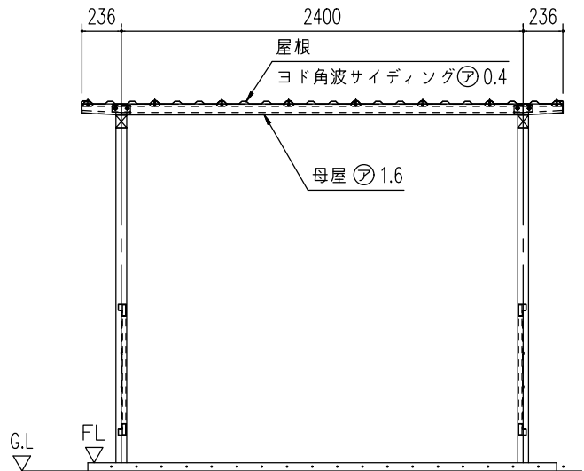
正面断面図 (S= 1/40)
