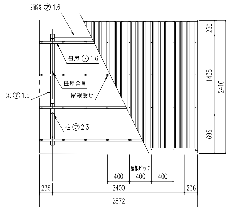
小 屋 伏 図 (S= 1/40)
