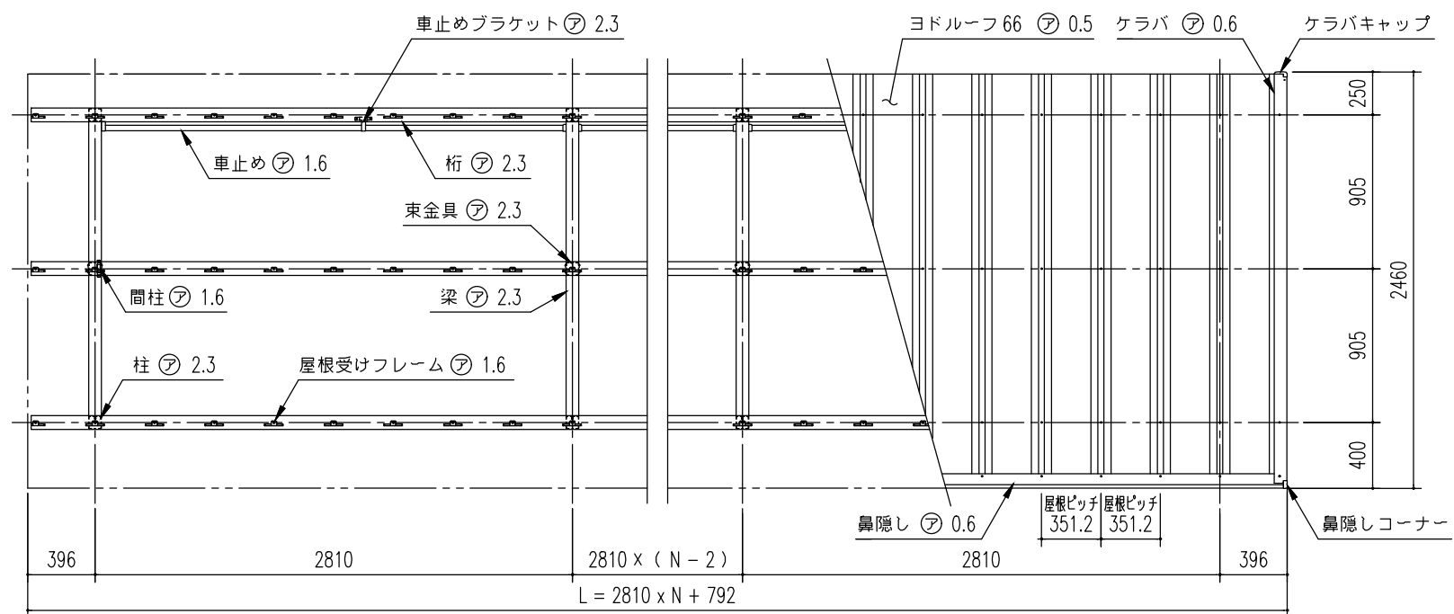
小屋伏図 (S=1/40)
