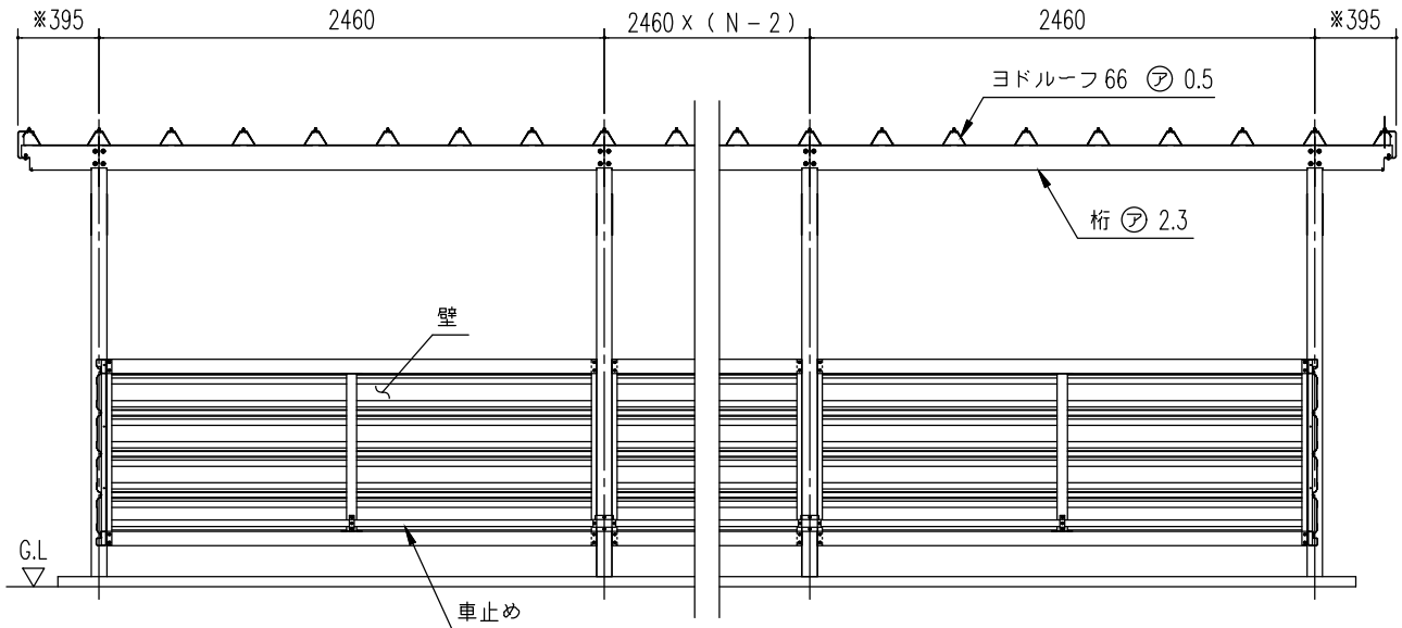
正面断面図 (S=1/40) （N：スパン数）
