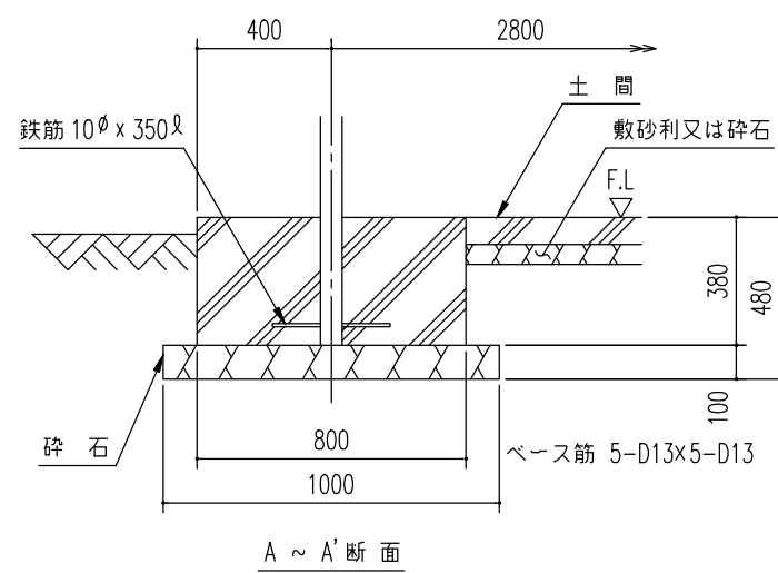
基礎断面図 (S=1/25) <下記条件での参考図> (地耐力 50 kN/m 2 以上, コンクリート設計基準強度 18 N/mm 2 以上) (基準風速 34 m/s, 地表面粗度区分 Ⅲ) 注1) 寒冷地の場合、凍結深度等を考慮し、実情にあわせて設計して下さい。 注2) その他現地の実情にあわせて設計して下さい。
