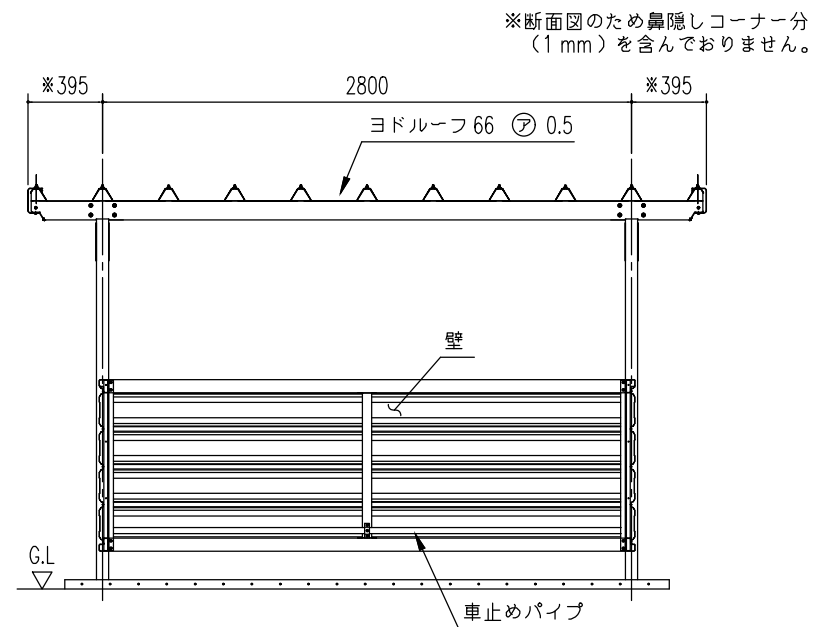
正面断面図 (S=1/40)
