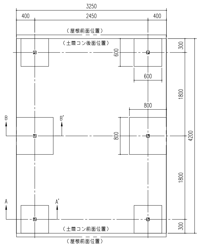
基礎伏図 (S=1/40)
