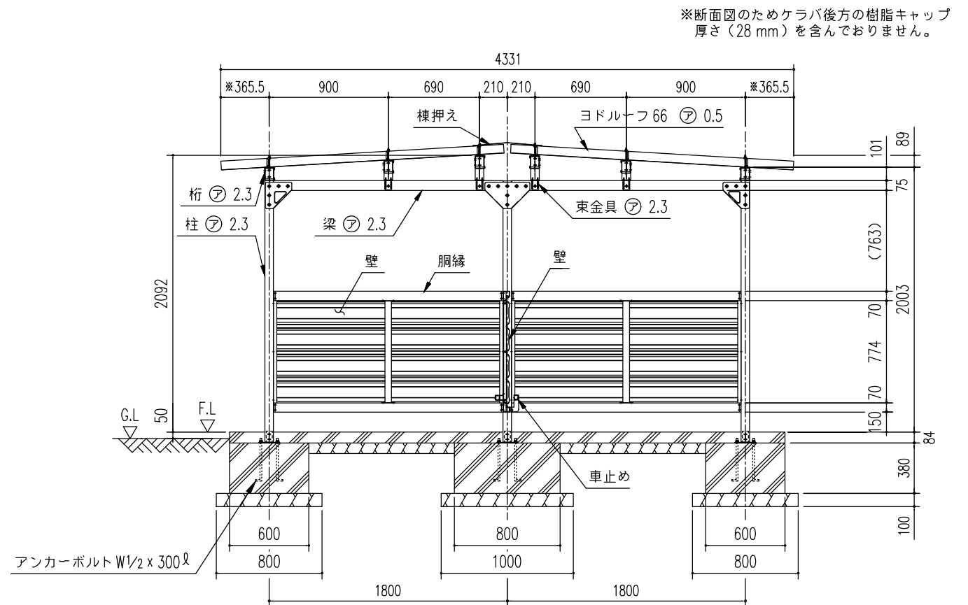
側面断面図 (S= 1/40)
