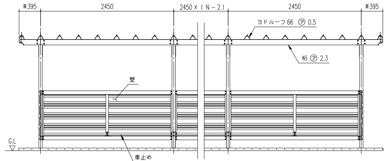
正面断面図 (S=1/40) （N：スパン数）
