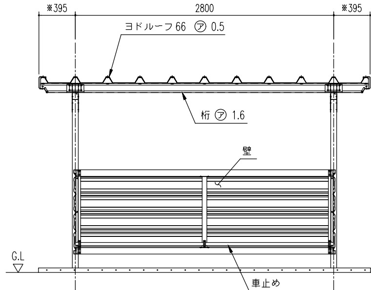
正面断面図 (S= 1/40)
