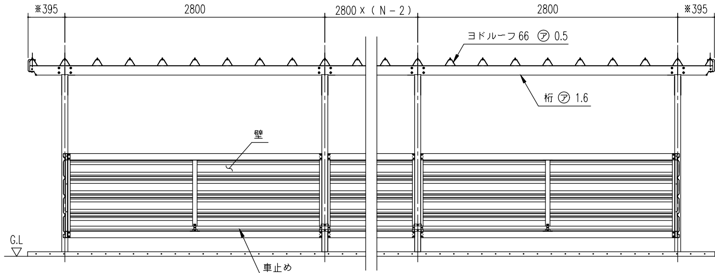
正面断面図 (S=1/40) （N：スパン数）
