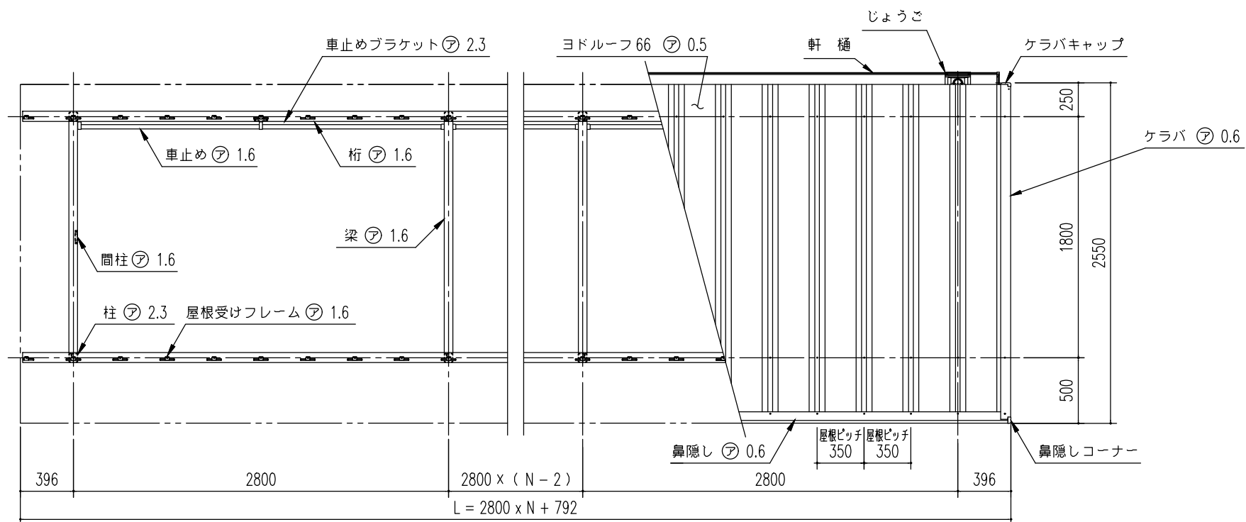
小 屋 伏 図 (S=1/40)
