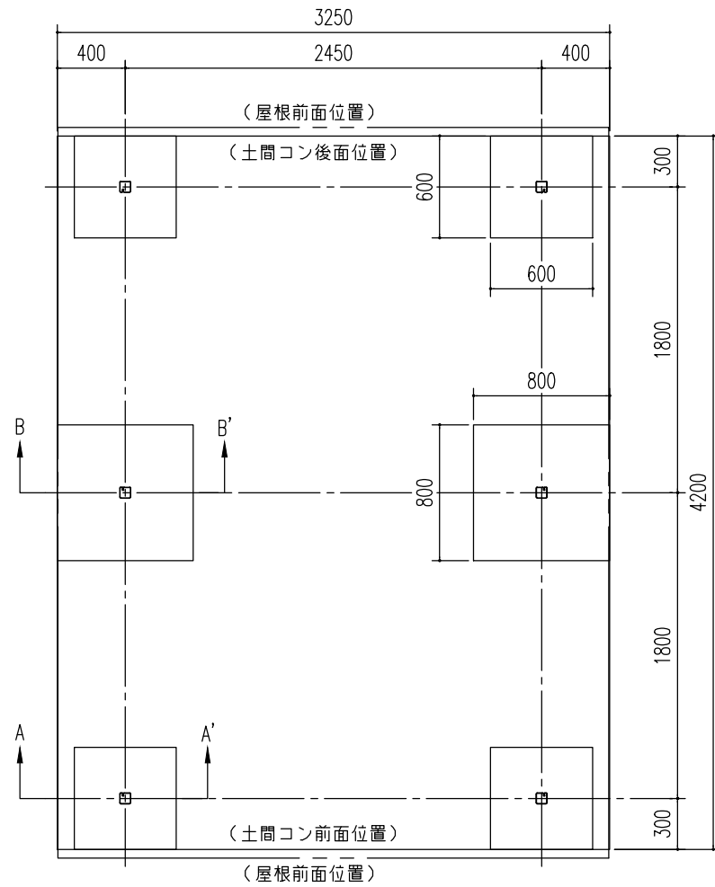
基礎伏図 (S = 1/40)
