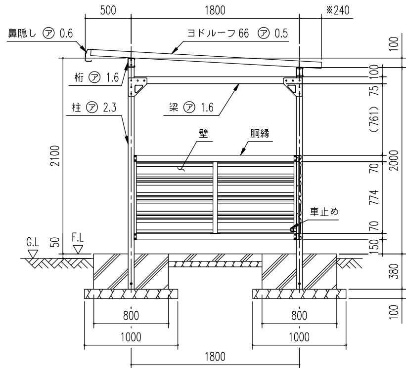
側面断面図 (S=1/40)
