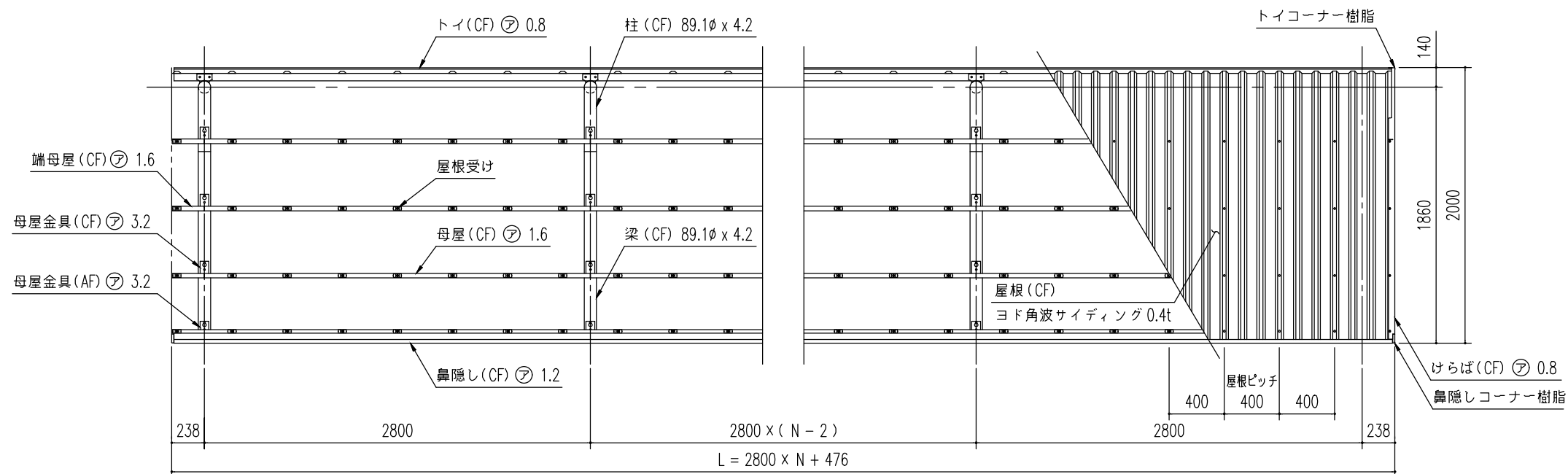
小屋伏図 (S=1/40) (N: スパン数)
