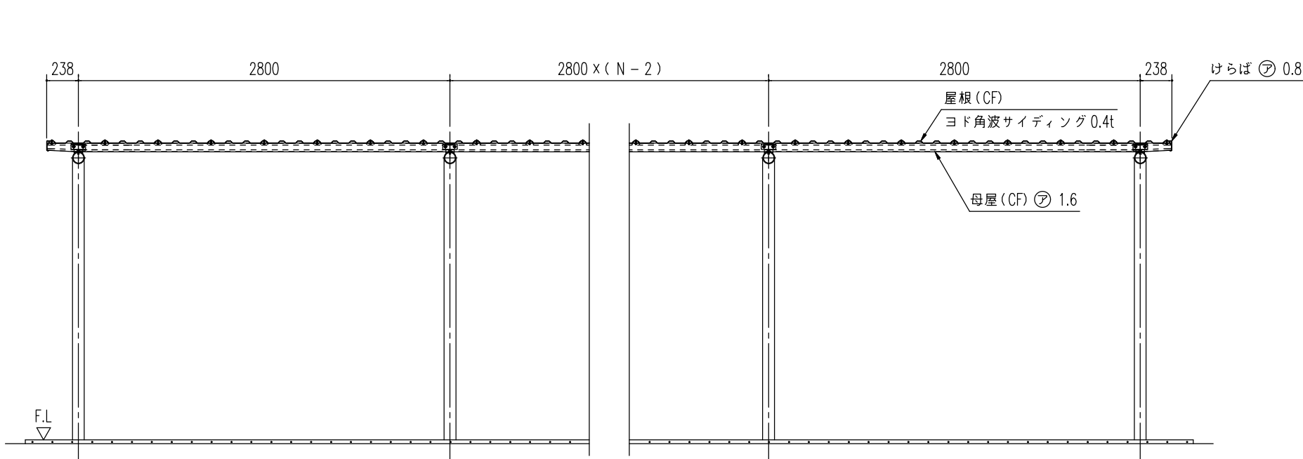
正面断面図 (S= 1/40) ( N : スパン数 )
