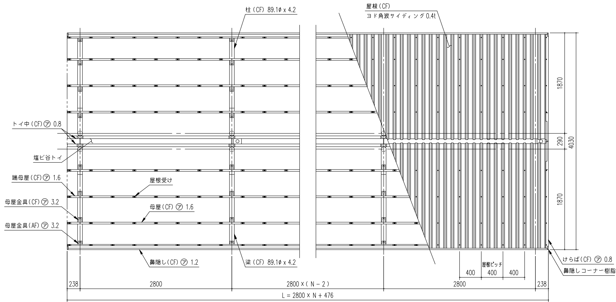
小 屋 伏 図 (S= 1/40)
