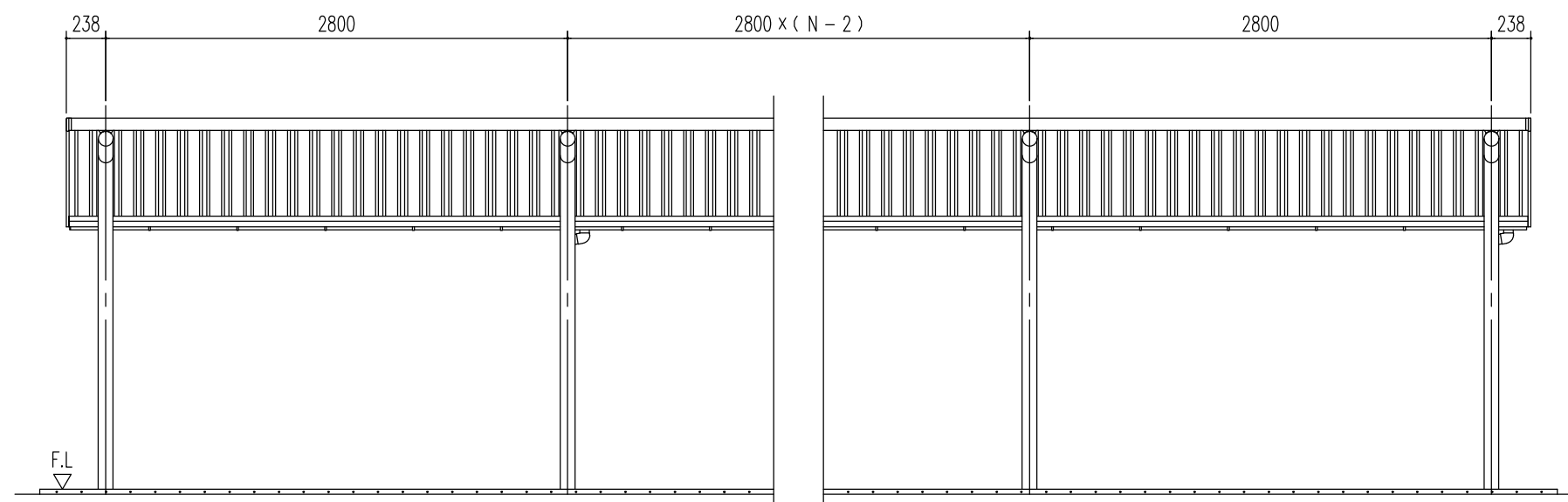
正 面 立 面 図 (S= 1/40) ( N : スパン数 )
