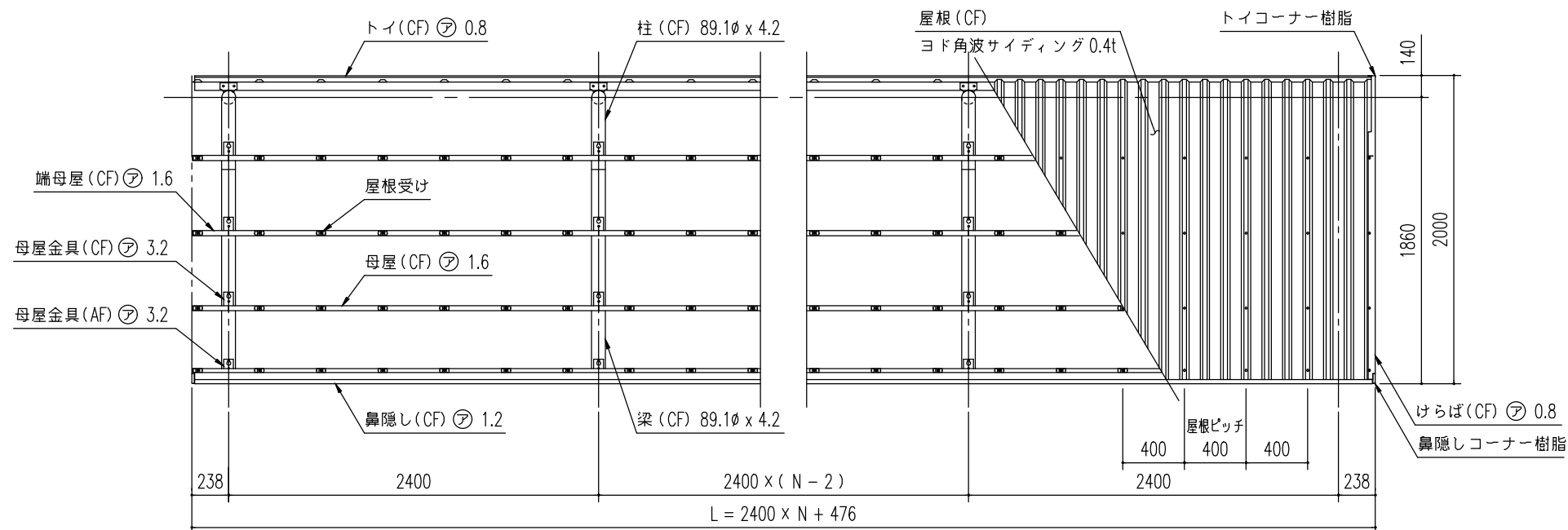
小屋伏図 (S= 1/40) ( N : スパン数 )
