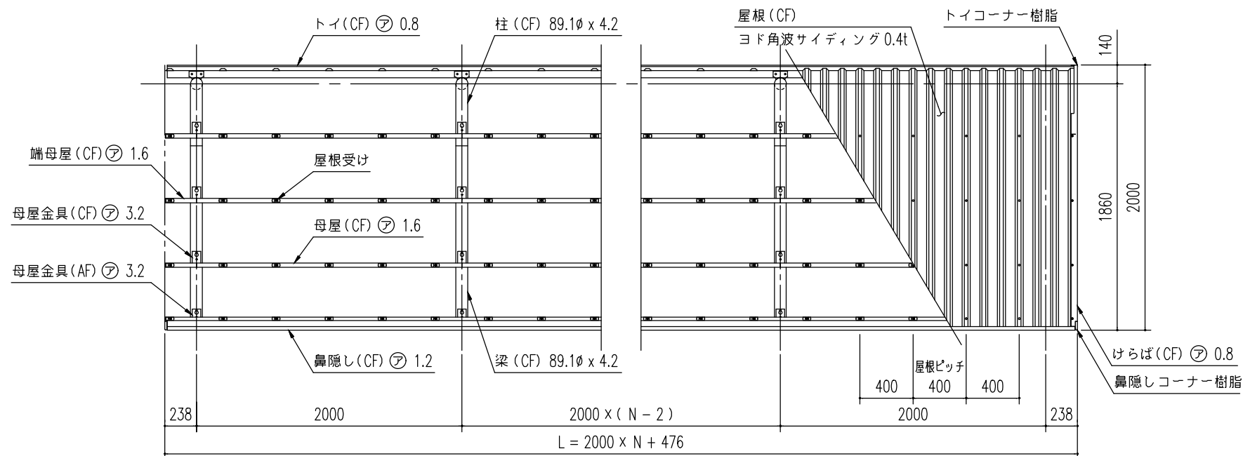
小屋伏図 (S=1/40) (N: スパン数)
