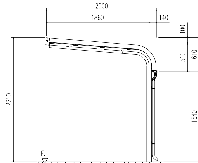
側面立面図 (S=1/40)
