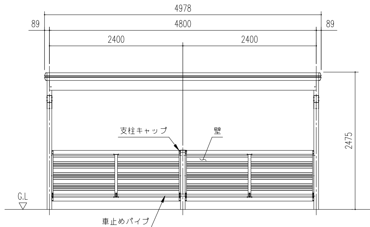
正面立面図 (S= 1/40)
