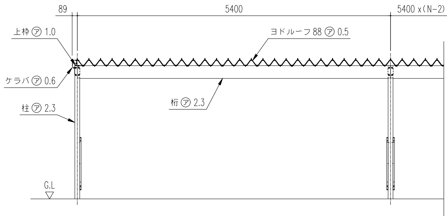
正面断面図 (S= 1/40)
