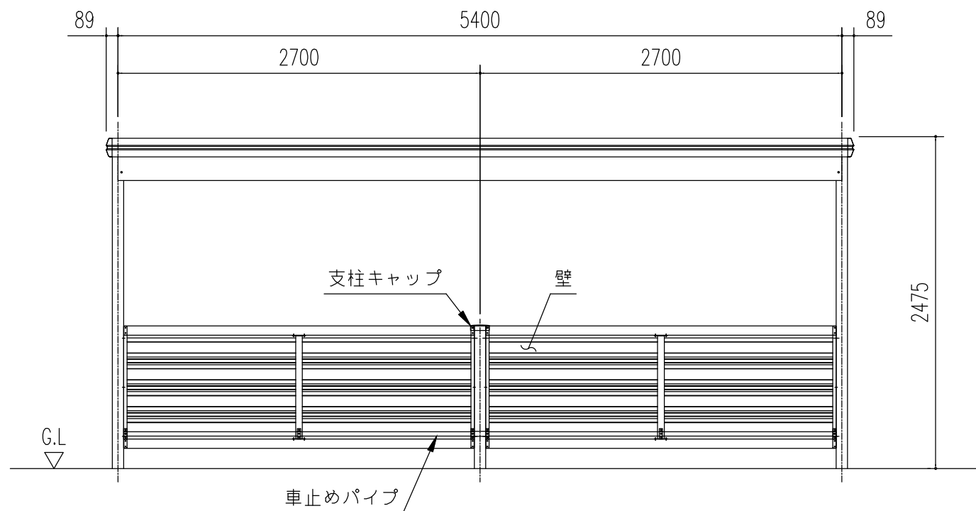
正面立面図 (S=1/40)
