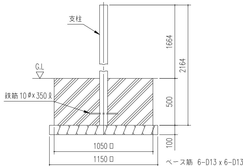
B 断面
