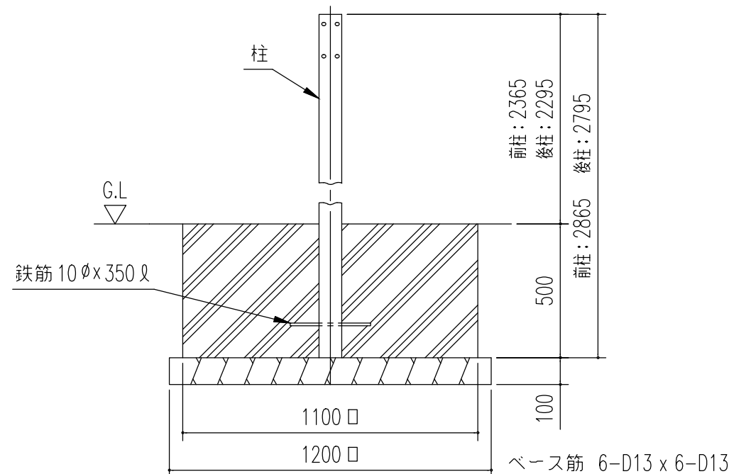
A 断面
