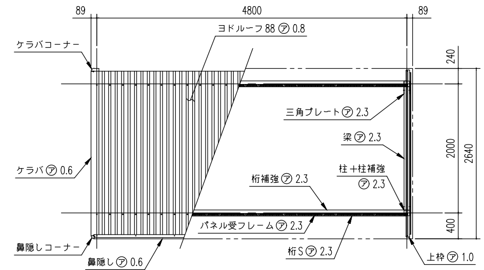
小屋伏図 (S= 1/60)
