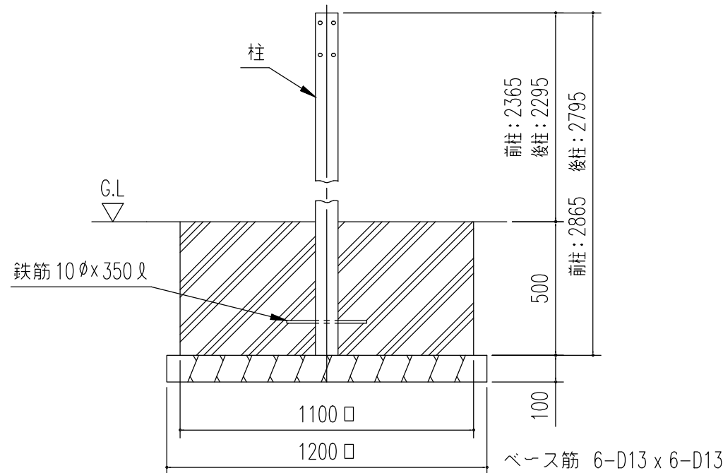
A 断面
