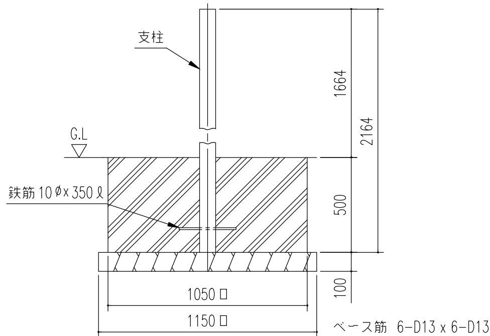
B 断面
