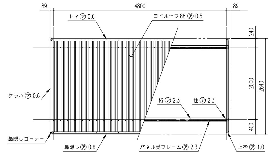
小屋伏図 (S= 1/60)
