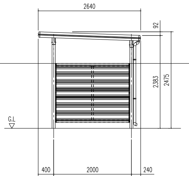
側面立面図 (S= 1/60)
