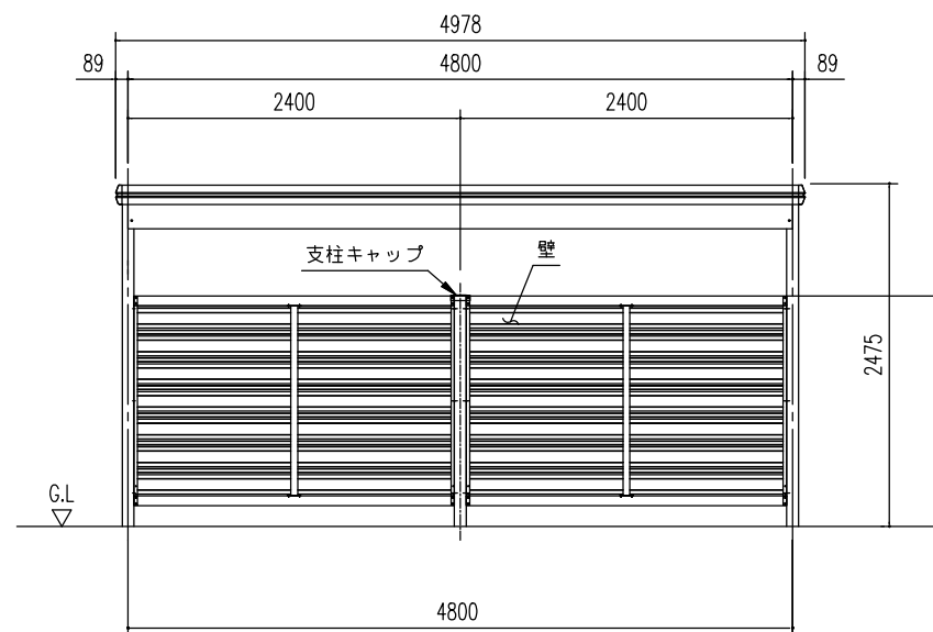
正面立面図 (S= 1/60)
