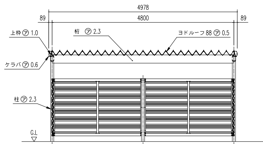
正面断面図 (S= 1/60)
