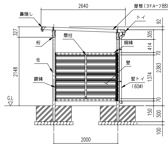
側面断面図 (S= 1/60)
