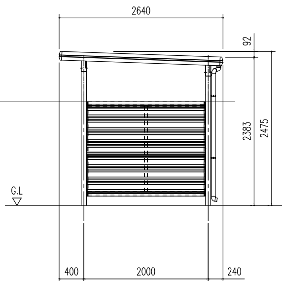
側面立面図 (S= 1/60)
