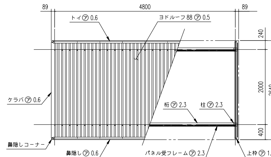
小屋伏図 (S= 1/60)
