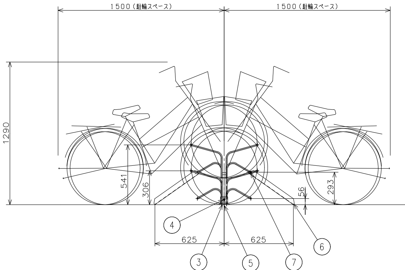
側面図 1:15
