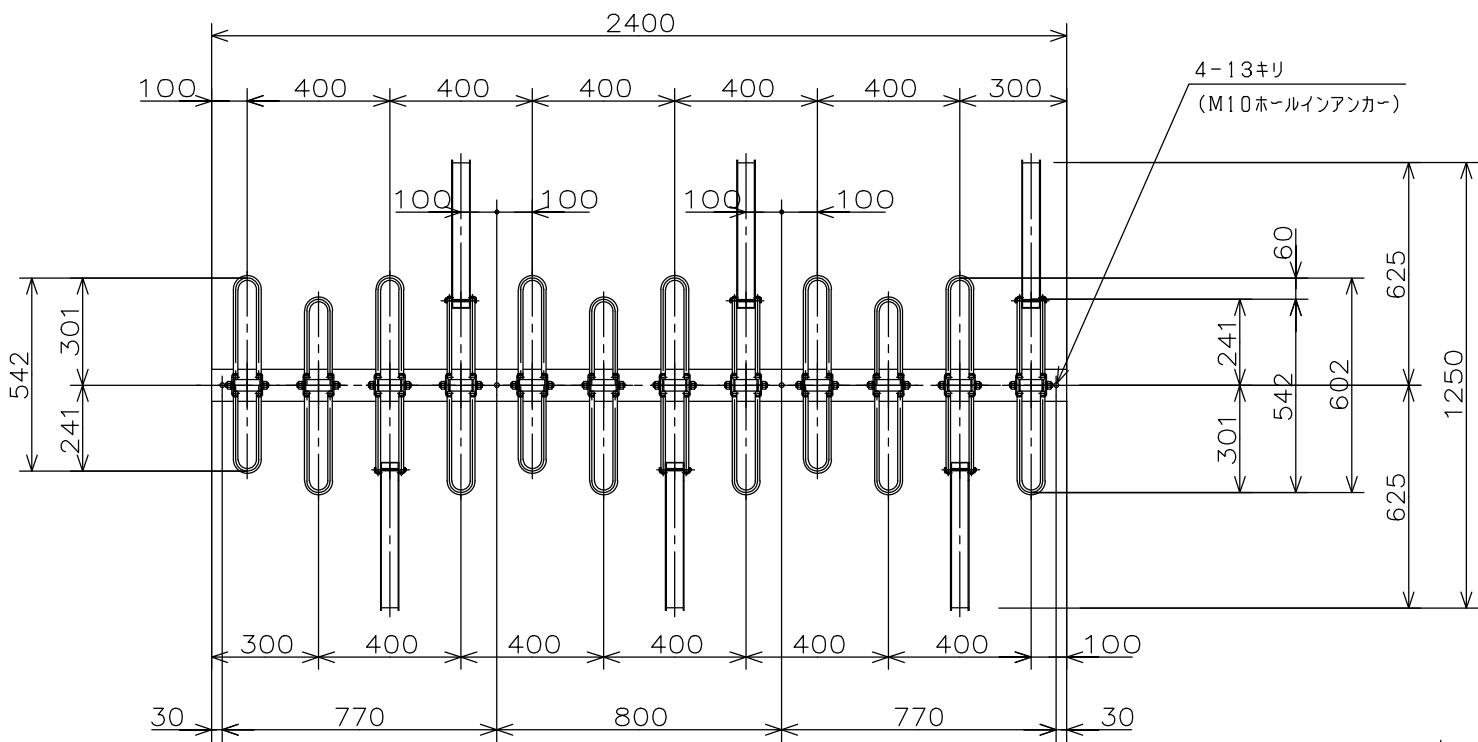
平面図 1:15
