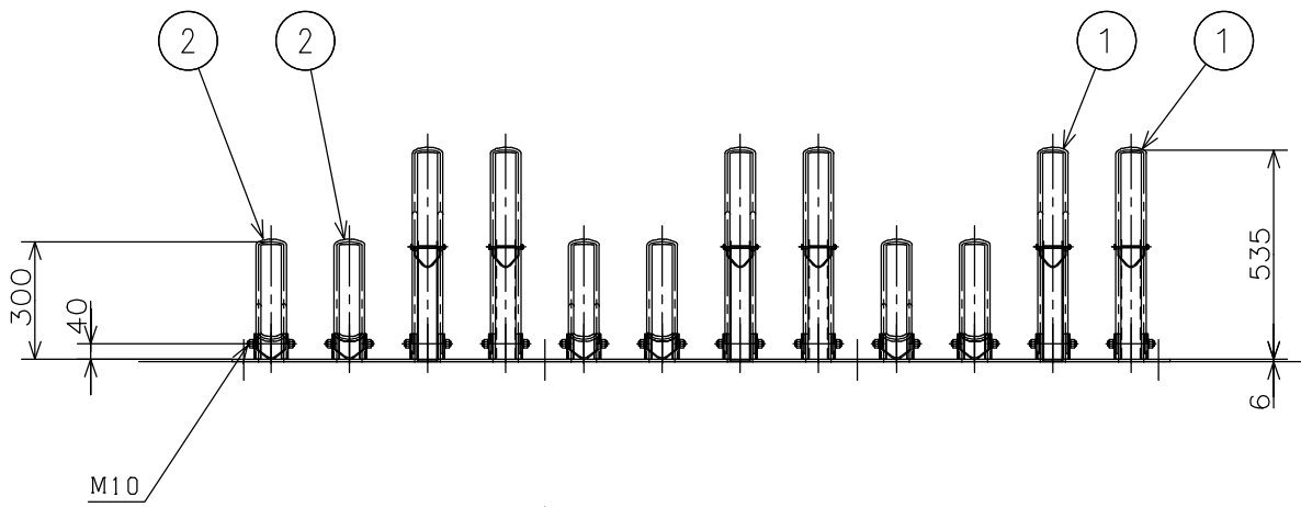
立面図 1:15
