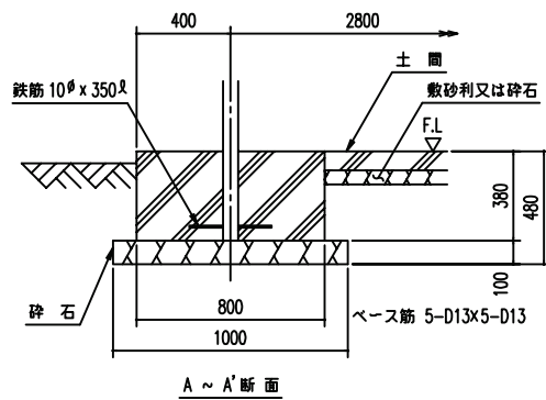
基礎断面図 (S=1/25)
