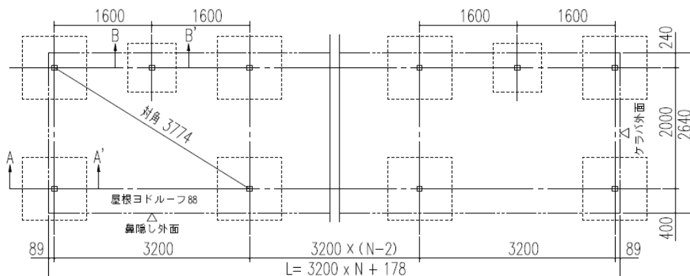
基礎伏図
