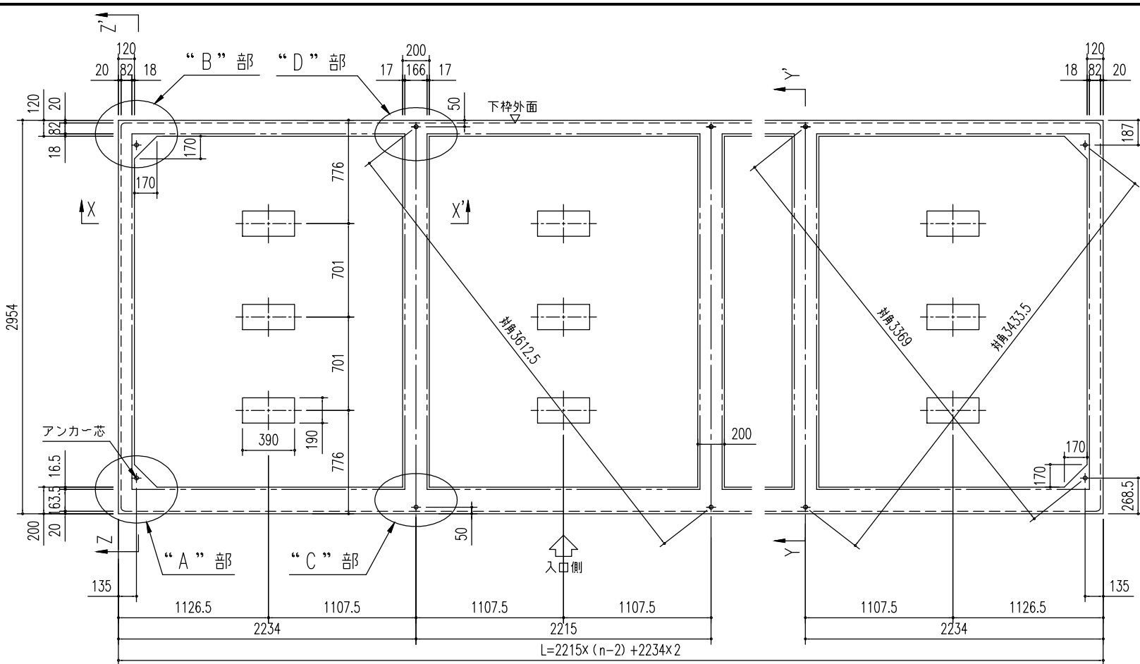
基礎伏図 (S=1/40)
