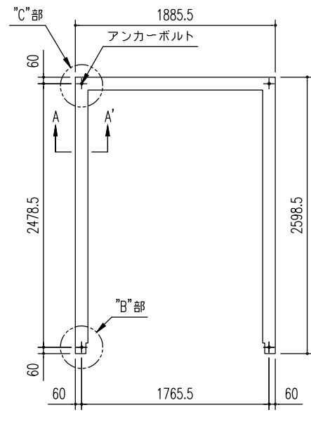
布基礎伏図 (s=1/50)
