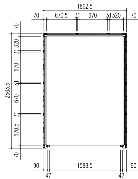
平面図 (s=1/50)
