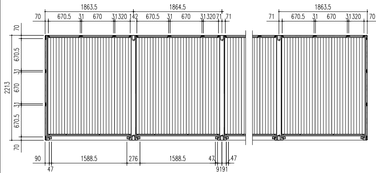
平面図 (S = 1/50)
