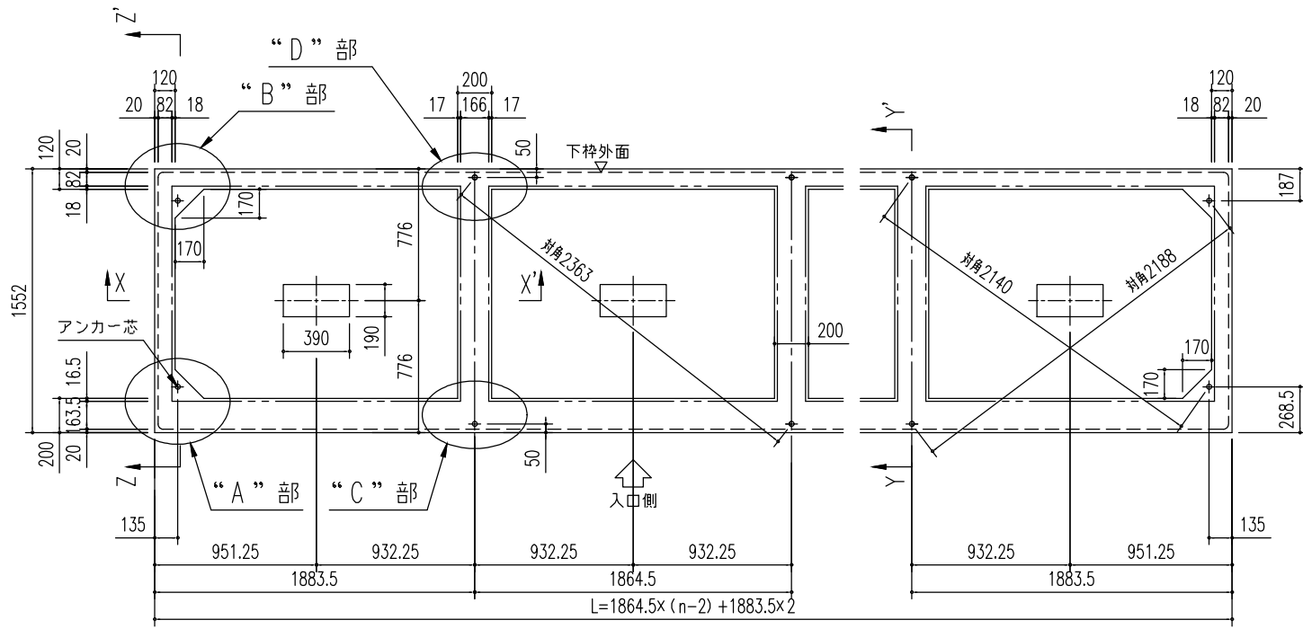
基礎伏図 (S=1/40)
