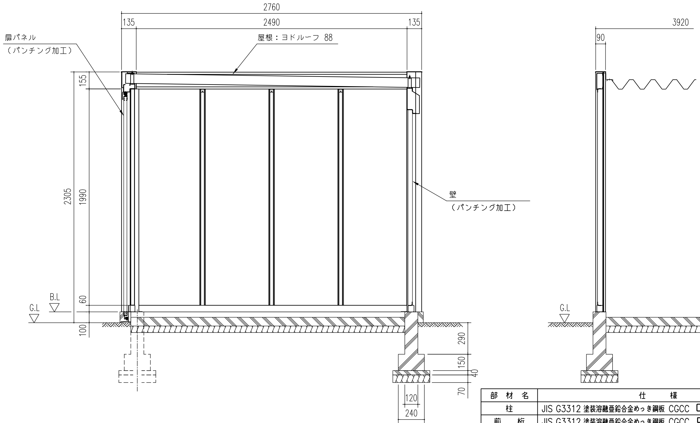
断面詳細図 縮尺=1/20
