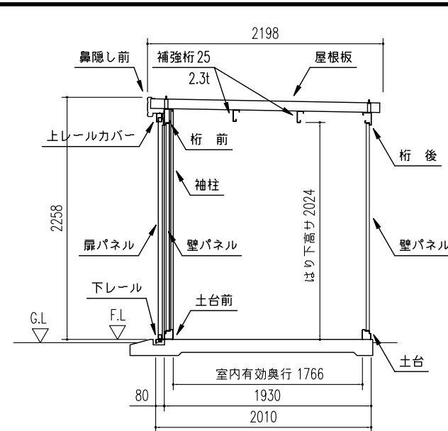
矩計図 (S=1/50)
