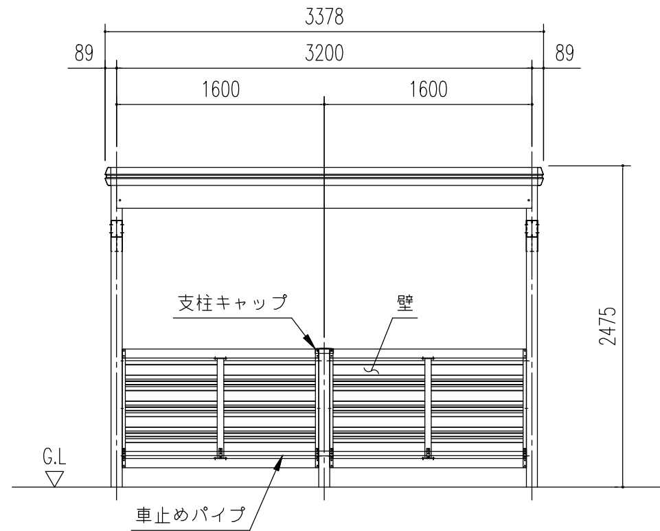
正面立面図 (S=1/40)
