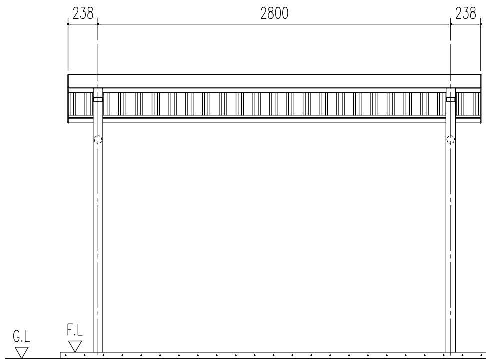
正面立面図 (S=1/30)
