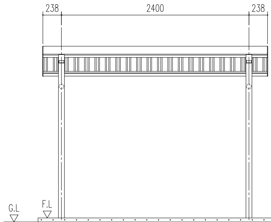
正面立面図 (S= 1/30)
