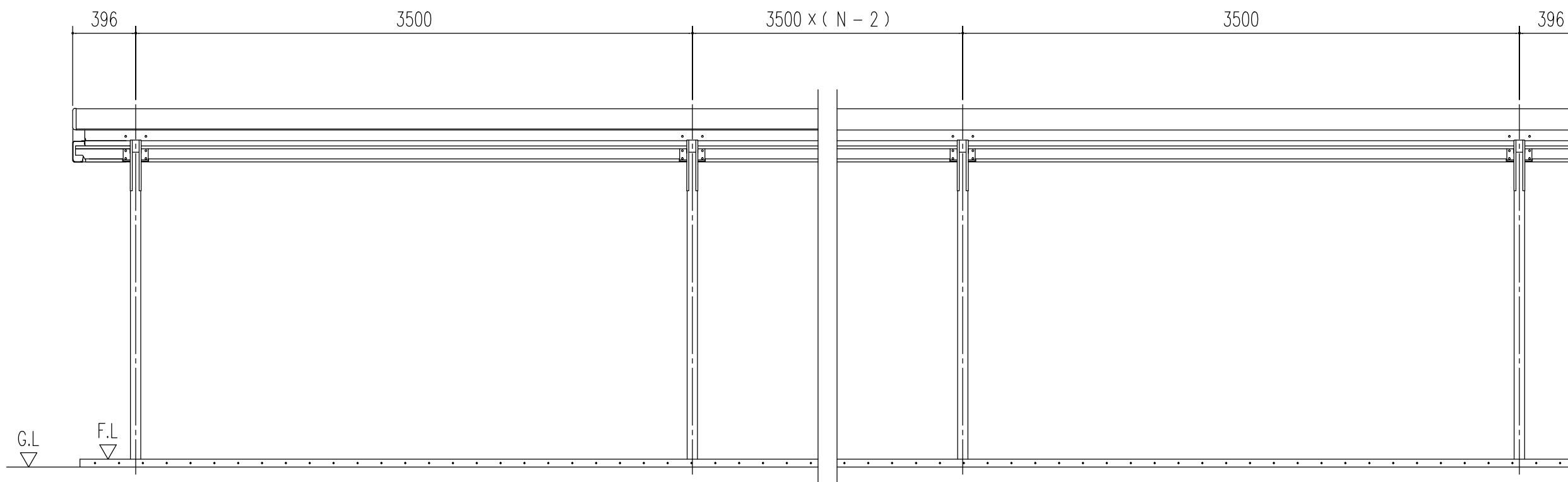
正面立面図 (S=1/30) (N: スパン数)
